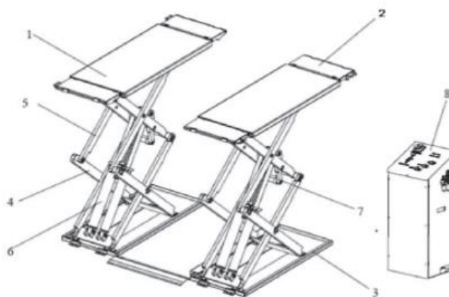
Рисунок 2.8 – Ножничный подъемник
