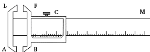
Рис.2. Схема штангенциркуля.
