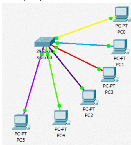
Рисунок 46 – Цветовая расцветка кабеля
