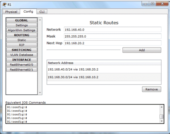
Рисунок 51 – Статическая маршрутизация 3) Настройка статической маршрутизации заключается в ручном вводе в таблицу маршрутизации всех маршрутов, которые не являются
