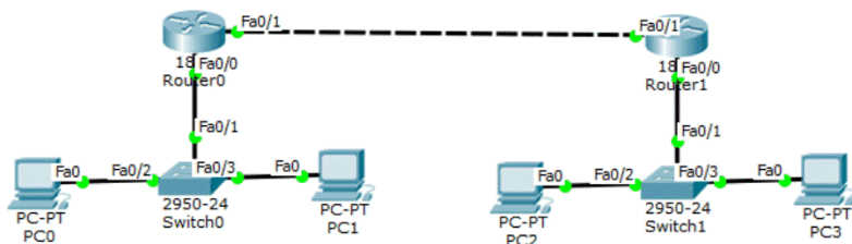
Рисунок 63 – Пример сети для поддержки IPv6 статической маршрутизации
