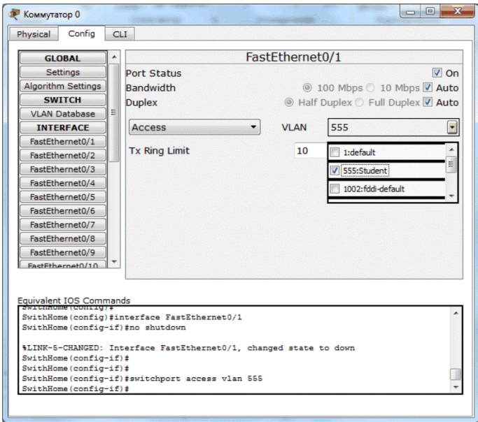
Рисунок 16 – Параметры интерфейсов коммутатора
