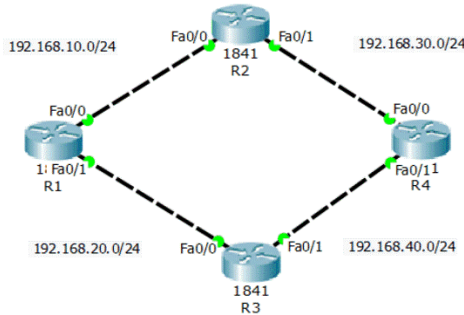
Рисунок 50 – Пример сети для настройки статической маршрутизации Таблица 2 – Назначение IP-адресов маршрутизаторов
