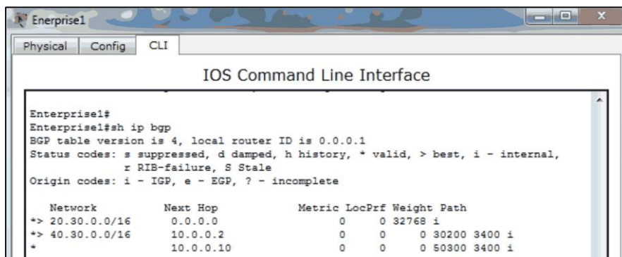
Рисунок 60 – Результат применение команды sh ip bgp
