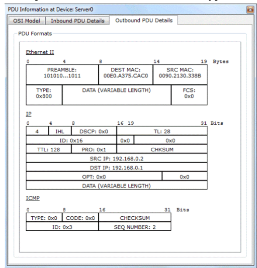
Рисунок 38 – Детализированная информация о исходящем пакете
