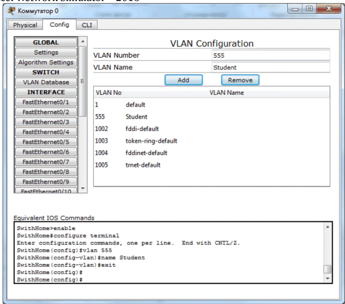
Рисунок 15 – База данных VLAN
