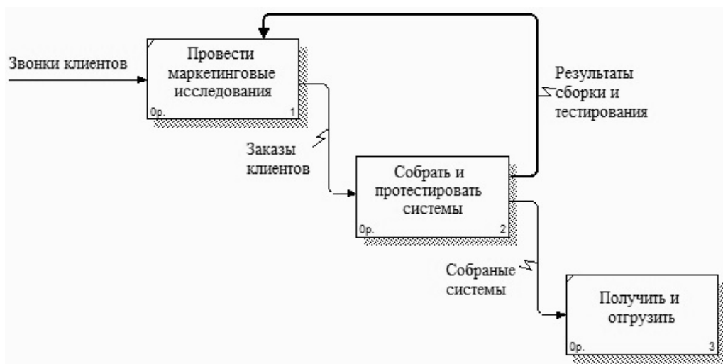
Рис. 26.4. Диаграмма FEO
