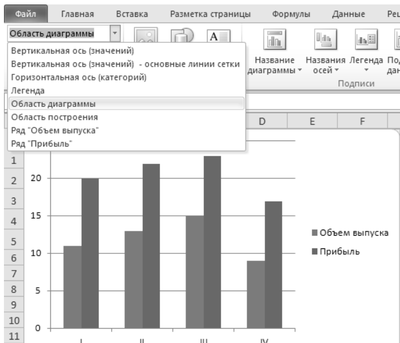
Рис. 4.3. Область диаграммы
