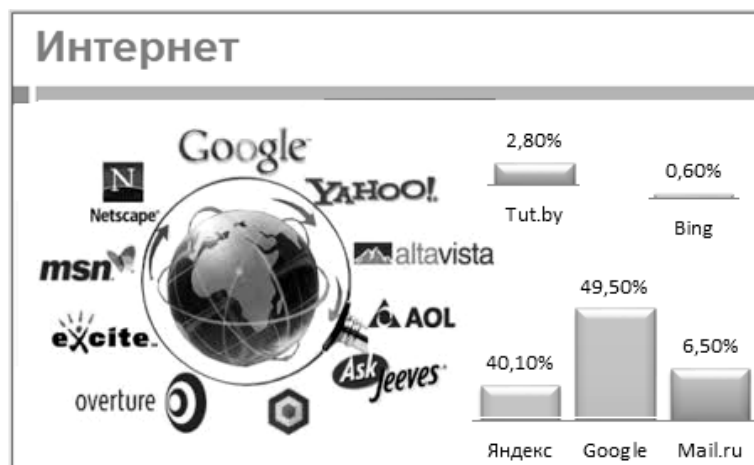
Рис. 6.10. Слайд № 9
