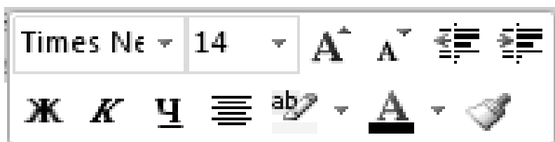
Рис. 2.1. Мини-панель инструментов
