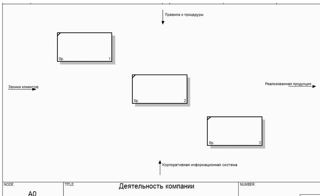
Рис. 24.3. Диаграмма декомпозиции
