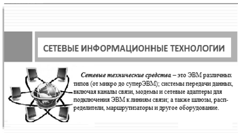
Рис. 6.4. Слайд № 4
