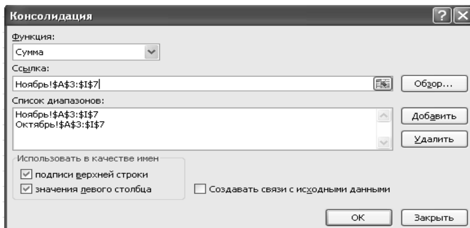
Рис. 5.59. Параметры консолидации
