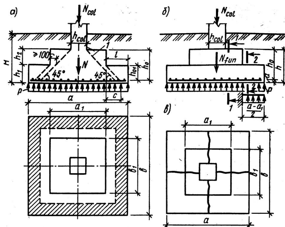
Рис. 2. К расчету отдельных центрально нагруженных фундаментов: 1 — пирамида продавливания
