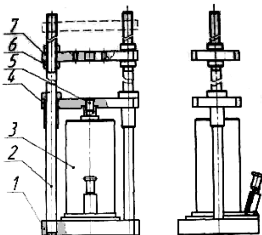
Рисунок 2.13– Гидравлический пресс
