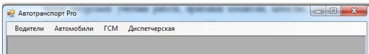
Рисунок 2.12 – Главная форма
