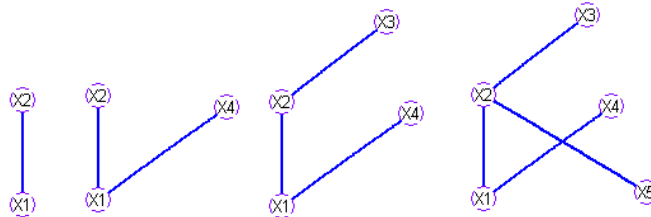
Рис.15. Ход построения минимального остовного дерева.
